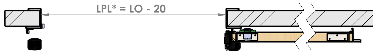
COUPE A-A
