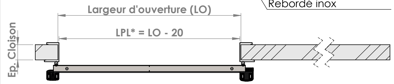
COUPE A-A
