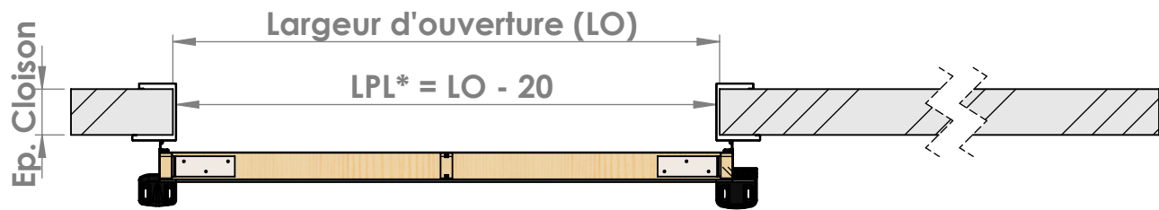
COUPE A-A
