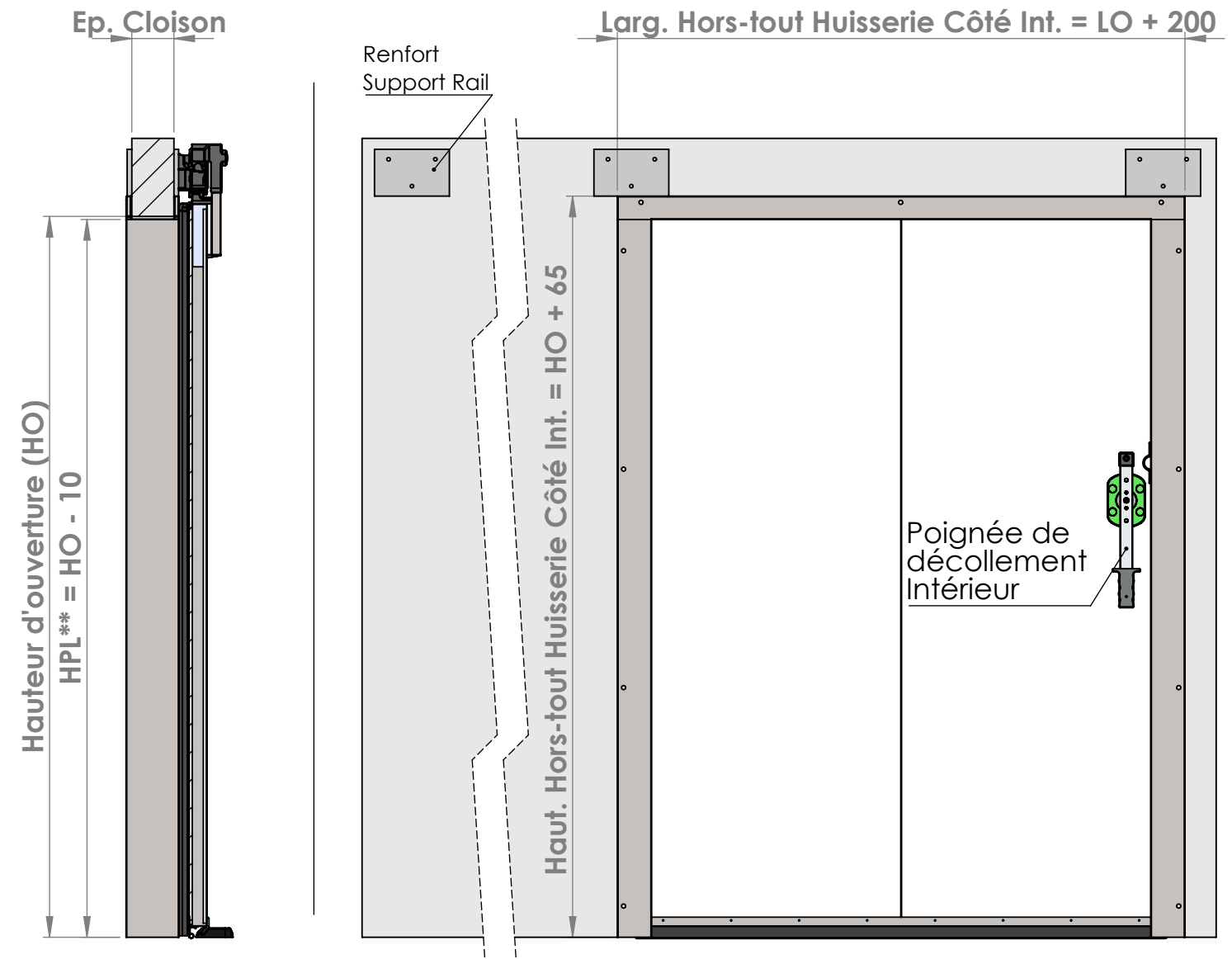
COUPE B-B
