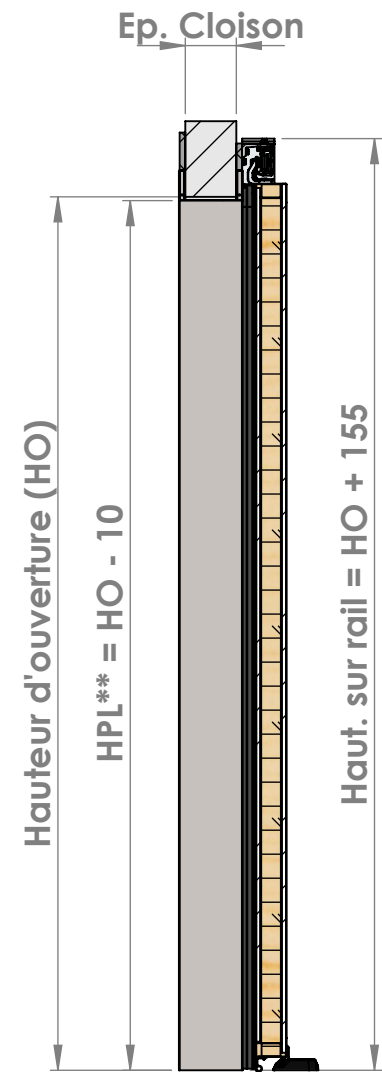
COUPE B-B
